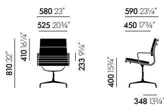
Soft Pad Chair EA 207 (nueva altura), no giratoria, con reposabrazos
