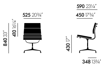
Soft Pad Chair EA 205 (altura clásica), no giratoria, sin reposabrazos
