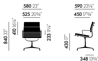
Soft Pad Chair EA 207 (altura clásica), no giratoria, con reposabrazos
