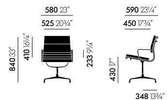
Soft Pad Chair EA 208 (altura clásica), giratoria, con reposabrazos
