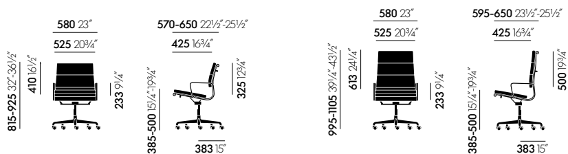
Soft Pad Chair EA 217, respaldo de altura media, giratoria, con reposabrazos
