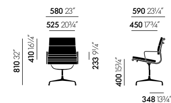
Soft Pad Chair EA 208 (nueva altura), giratoria, con reposabrazos
